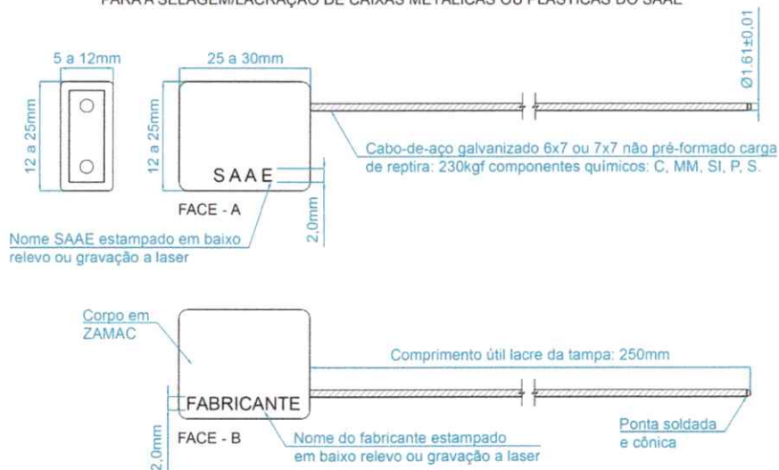
SELO (LACRE) DE SEGURANÇA METÁLICO DE CABO-DE-AÇO GALVANIZADO PARA A SELAGEM/LACRAÇÃO DE CAIXAS METÁLICAS OU PLÁSTICAS DO SAAE
