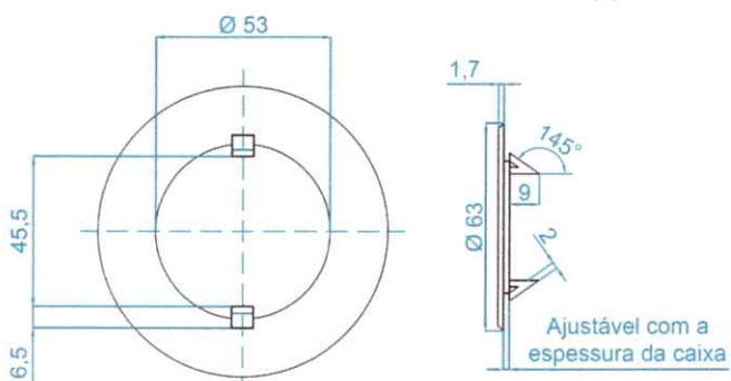
VEDANTE PARA FECHAMENTO DO FURO PARA TUBO CAMISA (1) E PARA FECHAMENTO DO FURO LATERAL (1)
