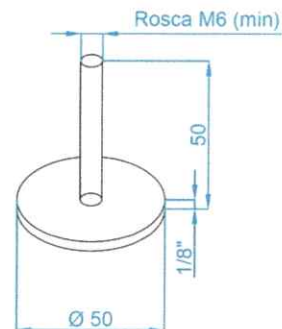
DETALHE DISPOSITIVO
