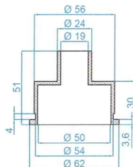
ACOPLADOR DE TUBO CAMISA
