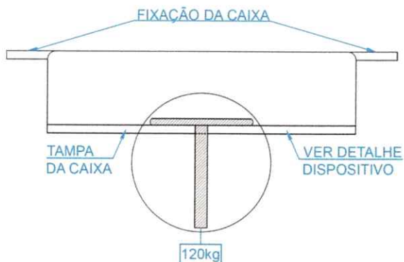
DESENHO ESQUEMÁTICO DO ENSAIO DE ARRANCAMENTO
